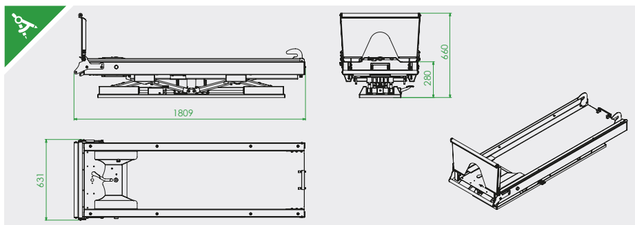
PA-555/2 FIJACION PARA CAMILLAS INOXIDABLE STRETCHER LOCKING SYSTEM SYSTÈME DE BLOCAGE DU BRANCARD INOX
