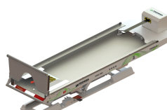
PA-490 SISTEMA DE CARGA ELÉCTRICA PARA BANCADAS ELECTRICAL LOADING SYSTEM FOR STRETCHER SUPPORT SYSTÈME DE CHARGEMENT ÉLECTRIQUE POUR SUPPORT DE BRANCARD
