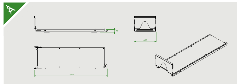
PA-555/2 FIJACION PARA CAMILLAS INOXIDABLE STAINLESS STEEL STRETCHER LOCKING SYSTEM SYSTÈME DE BLOCAGE DU BRANCARD INOX
